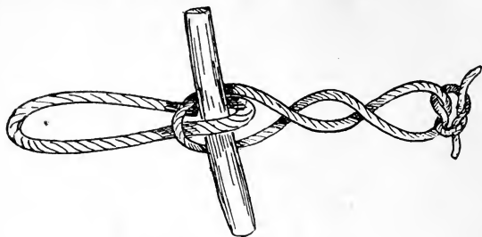
FIG. 144.—Rope buckle.
